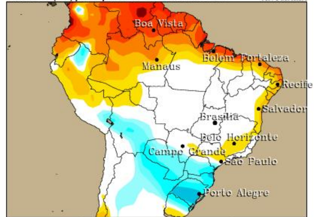
Prec ACUM (mm) para o período 01/07/2019 a 31/07/2019 ANOMALIA
