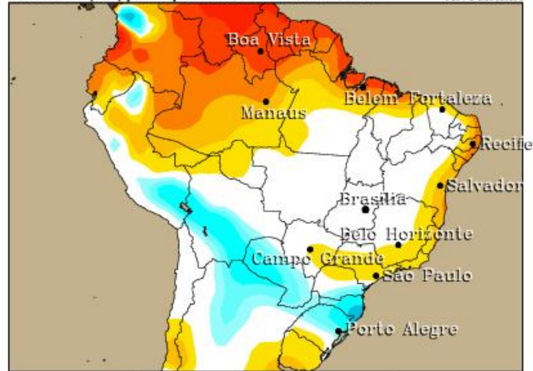
Prec ACUM (mm) para o período 01/08/2019 a 31/08/2019 ANOMALIA
