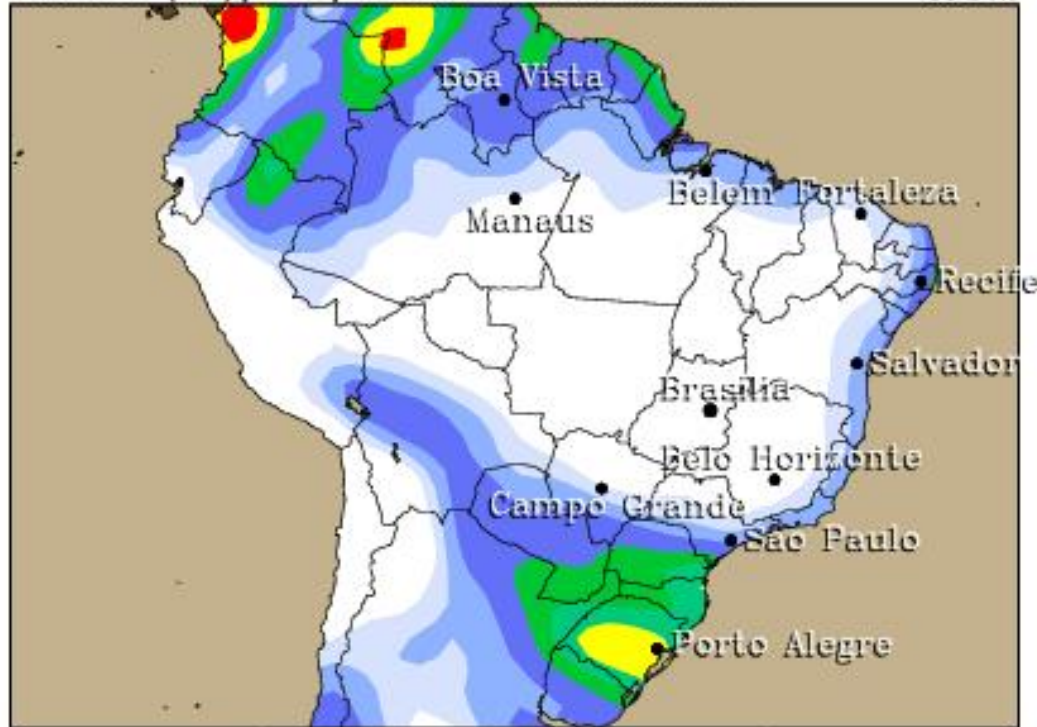
Prec ACUM (mm) para o período 01/07/2019 a 31/07/2019 CFSv2
